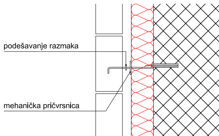
A-A presjek
